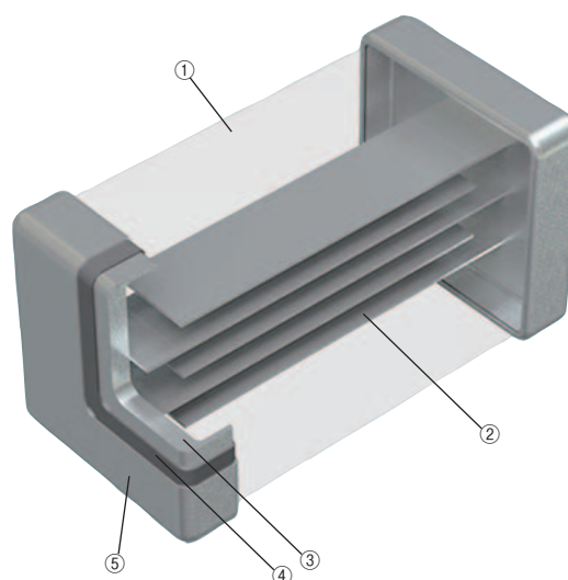
图2 积层芯片热敏电阻的内部结构
